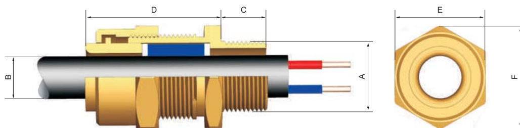
Cable wiring
